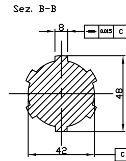
Albero UNI 8953 8x42x48 F
