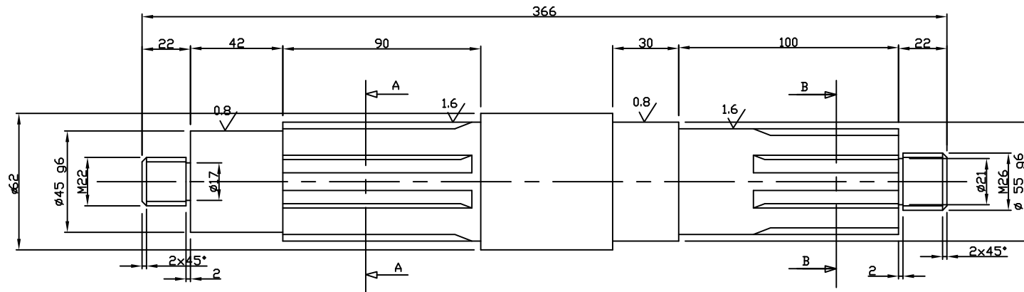
Albero UNI 8953 8x42x48 F
