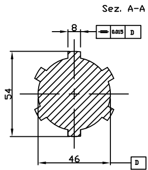
Albero UNI 8953 8x46x54 F
